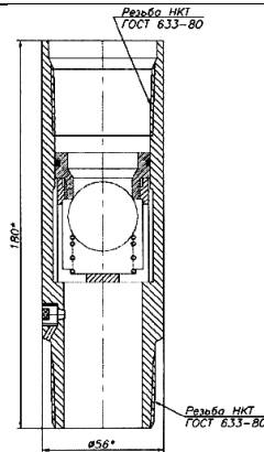
Вариант с винтом (сброс наружу)
