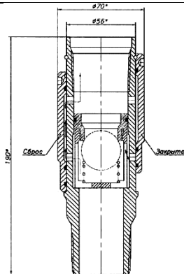
Вариант с золотником (сброс внутрь колонны)
